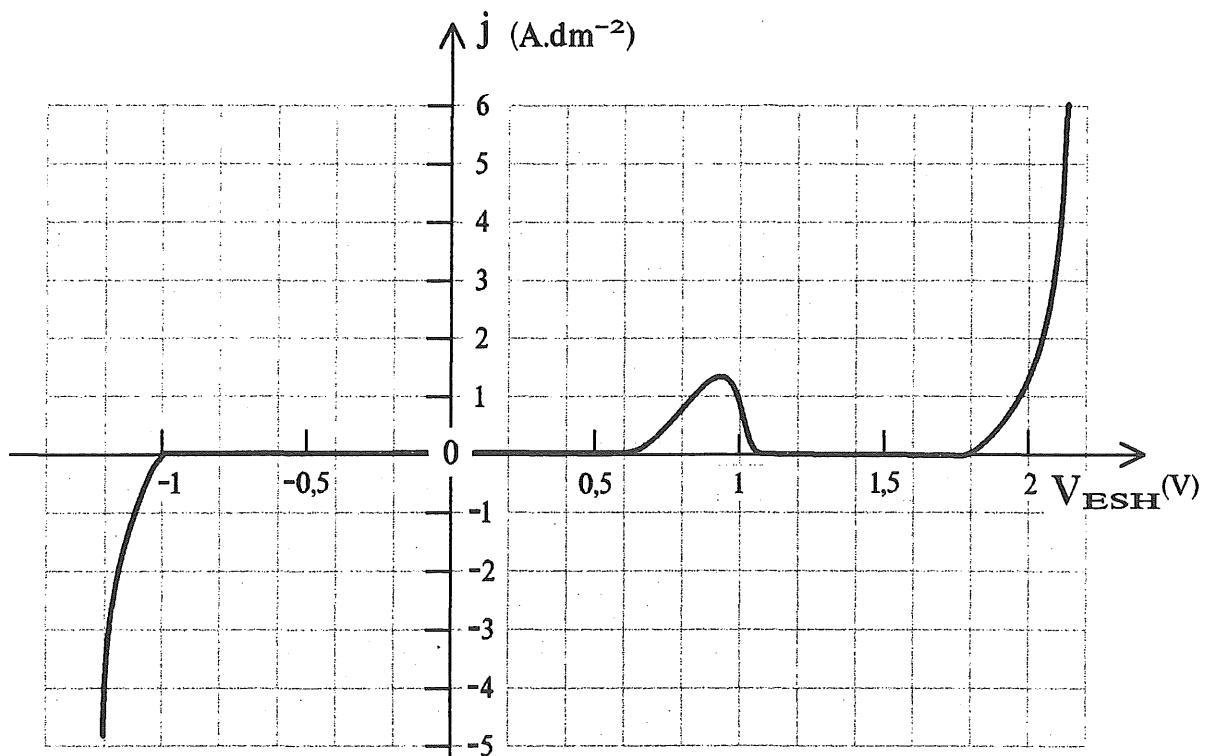
Figure 5. : Electrode de plomb
