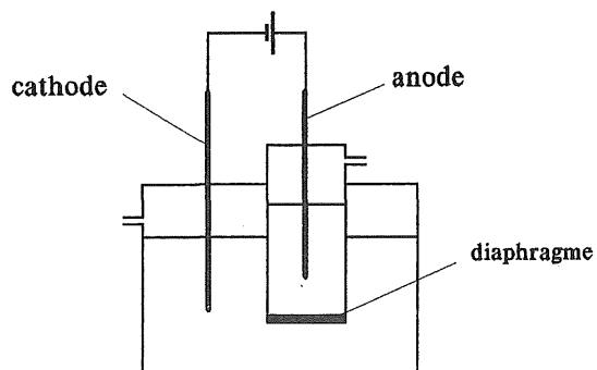
Figure 3 : Schéma de l'électrolyseur
