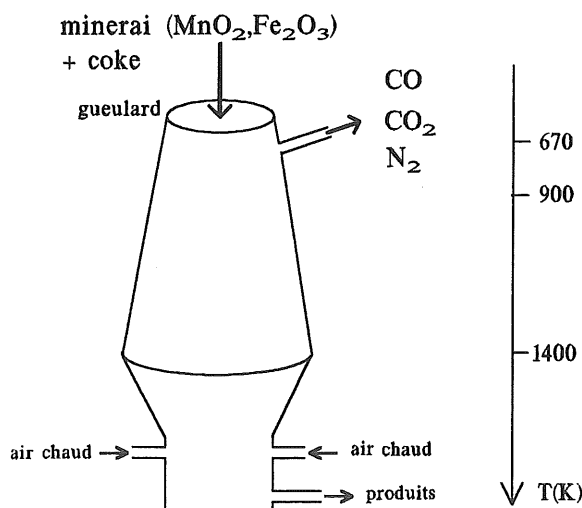
Figure 1. : Haut-fourneau à ferromanganèse
