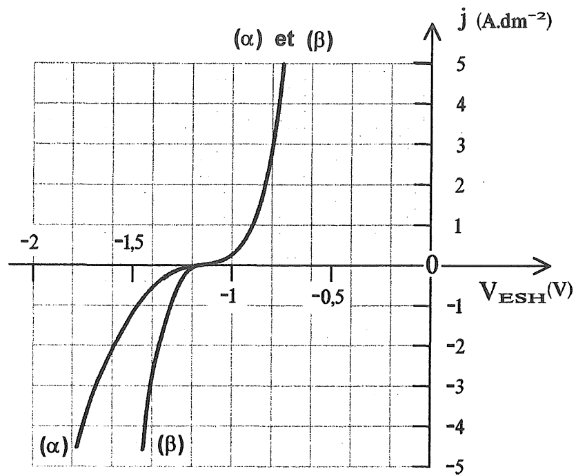
Figure 4. : Electrode de manganèse
